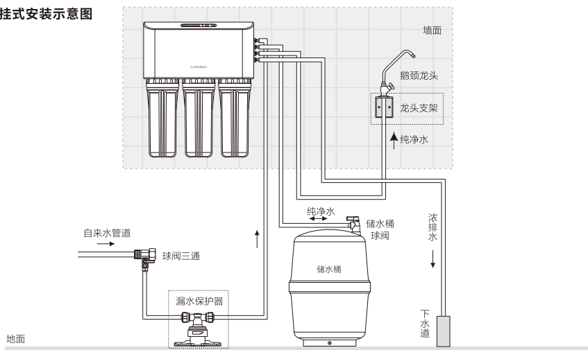
壁挂式安装示意图
